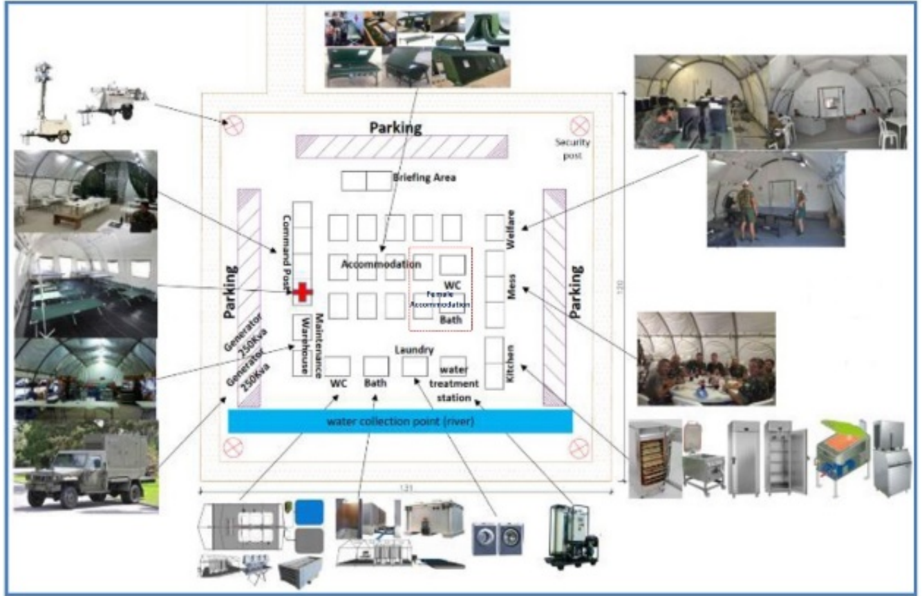
الشكل رقم ٦ نموذج قاعدة عمليات مؤقتة
